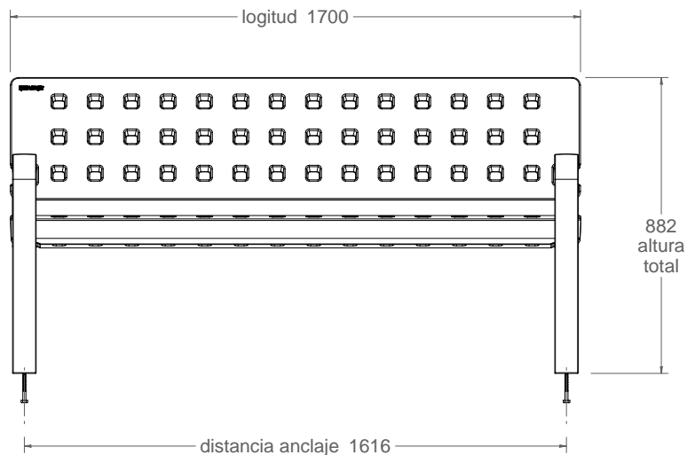
vista frontal 1:20
