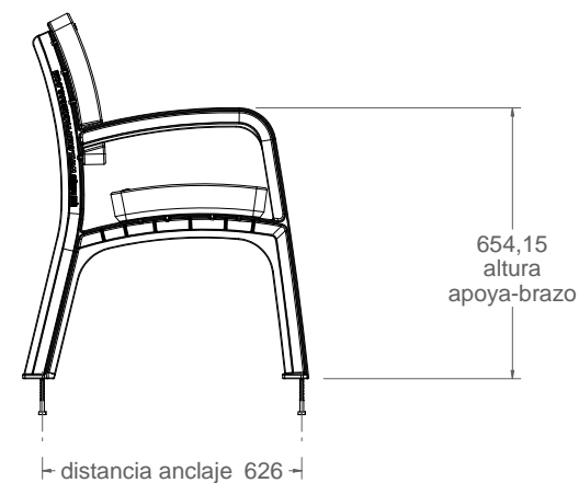
vista lateral 1:20
